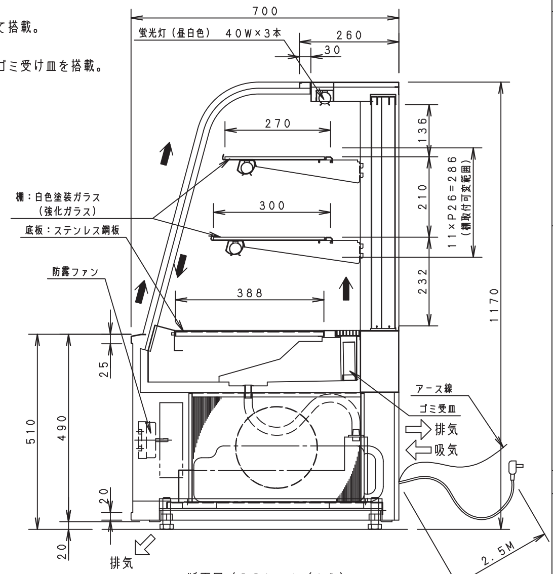
断面図 (SCL 1/10)
