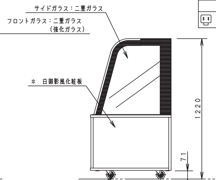
φ75自在キャスター
