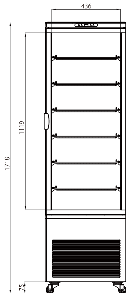
正面
