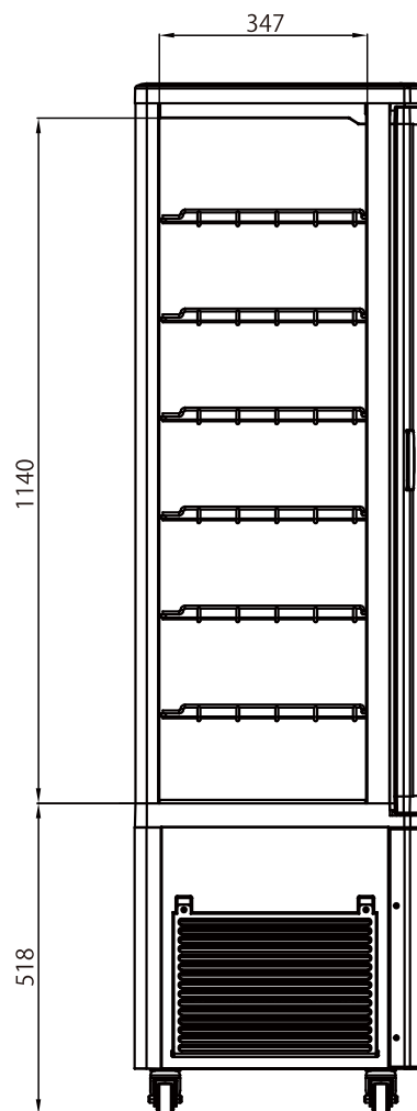
側面
